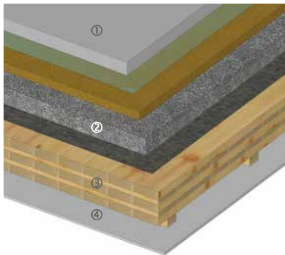
Abb. 45 Systemzeichnung einer gesamten Deckenkonstruktion mit Brettsperrelementen
