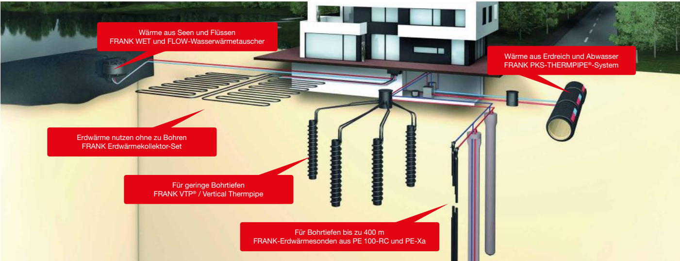
Zur Nutzung der Energie aus der Erde bietet das FRANK GET-System verschiedene Möglichkeiten zur sauberen und zukunftssicheren Wärmeenergiegewinnung
